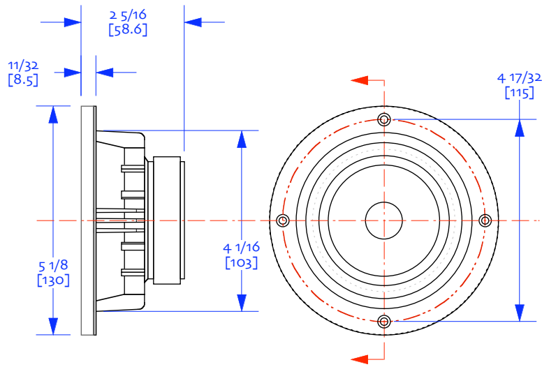
A: 1 magnet / no bezel cover
